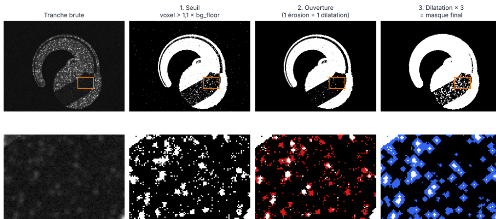
Canal DAPI, coupe z = 56 (jeu de démonstration). Ligne du bas : zoom sur la zone encadrée. rouge : voxels retirés - bleu : voxels ajoutés
