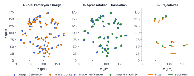
▲ La stabilisation : une rotation + translation (sans déformation) superpose les cellules de deux instants.
